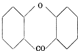
Xanthon.
